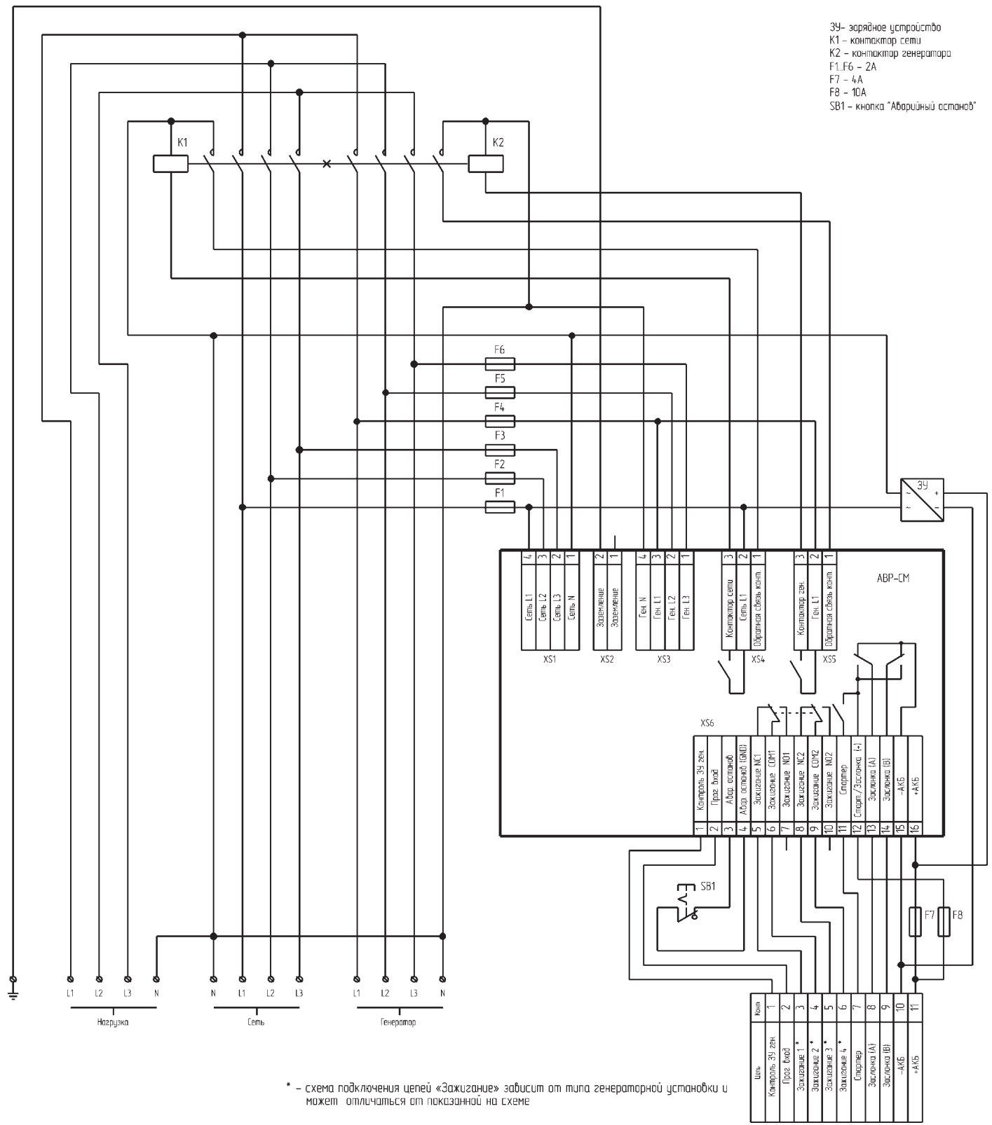
Рис. 6.2. Схема подключения АВР-СМ для конфигурации АВР33 с общим нейтральным проводом
